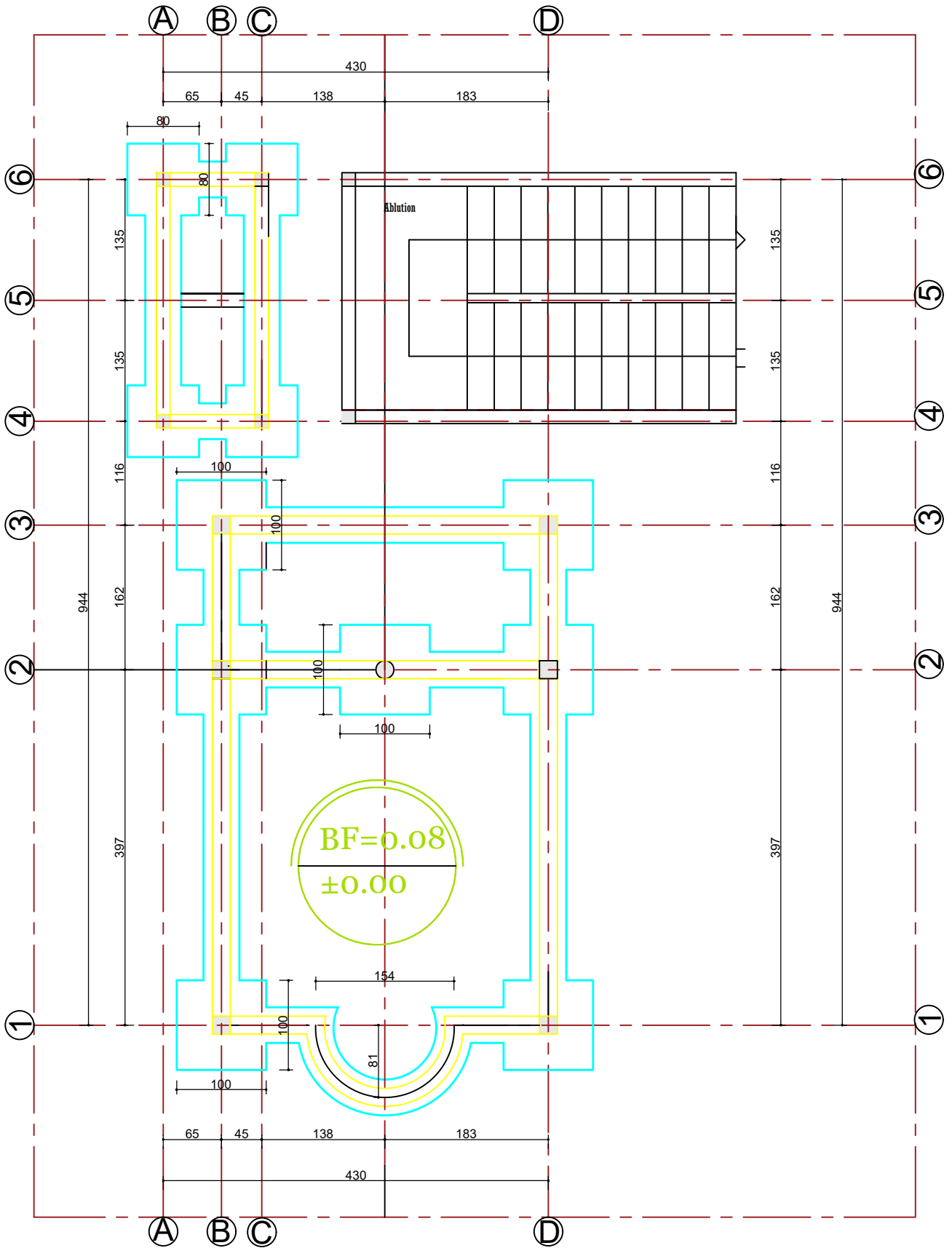
PLAN DE FONDATION
